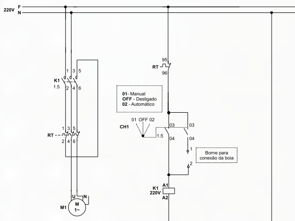
220V TRIFÁSICO
