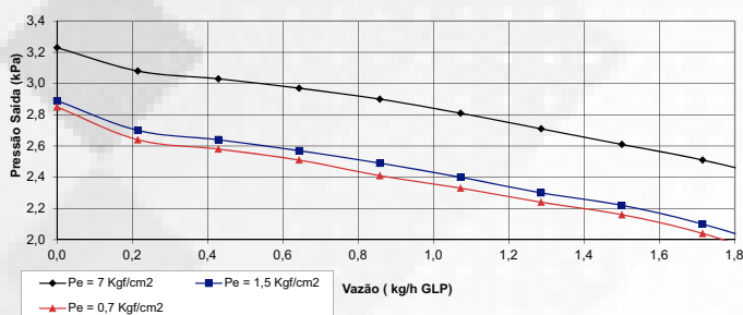
Gráfico de Desempenho Regulador 503 Ajuste: PE= 7 kgf/cm 2 PS= 2,8 kPa Vazão = 1 kg/h GLP
